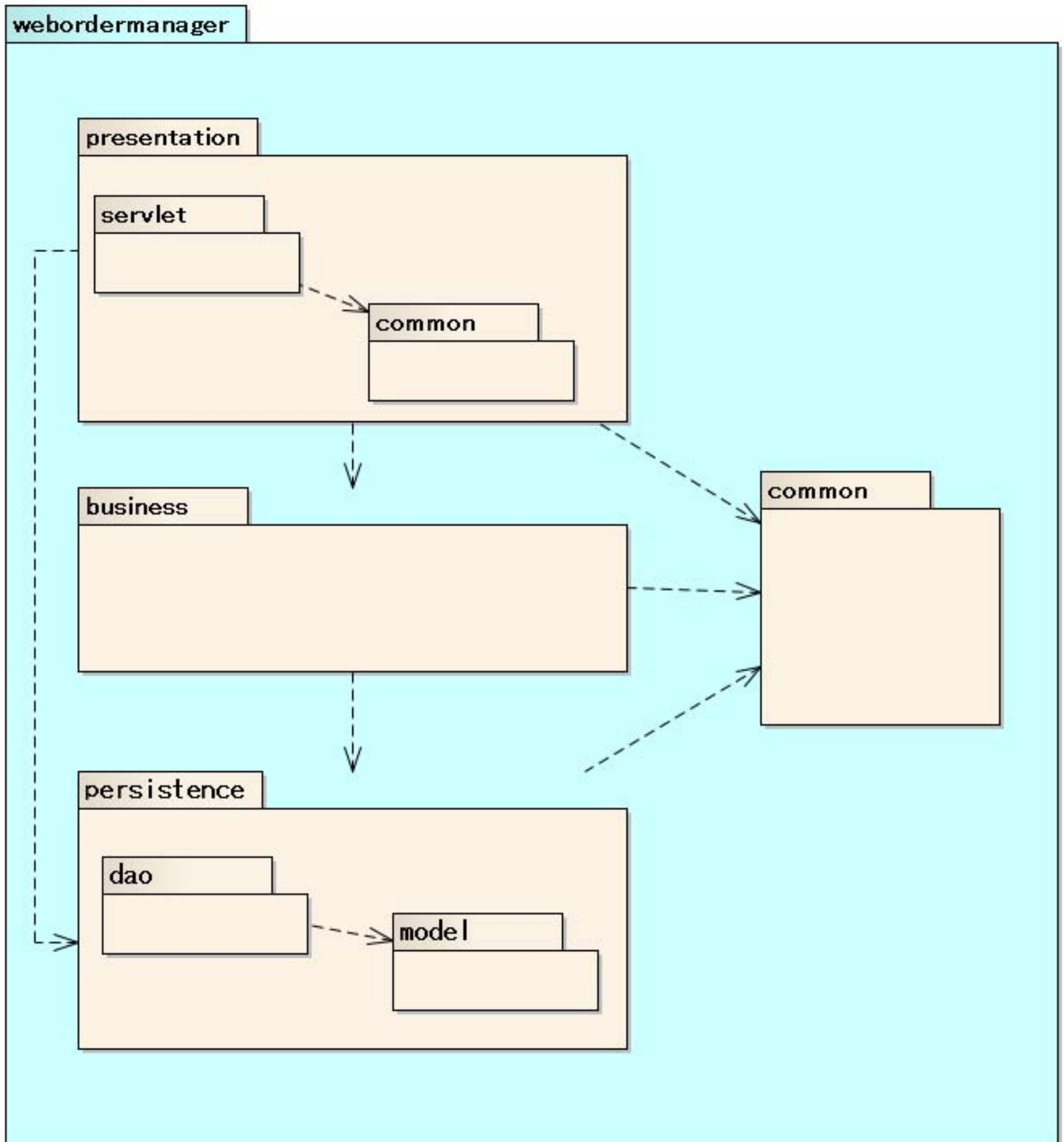
アプリケーション物理構造図
